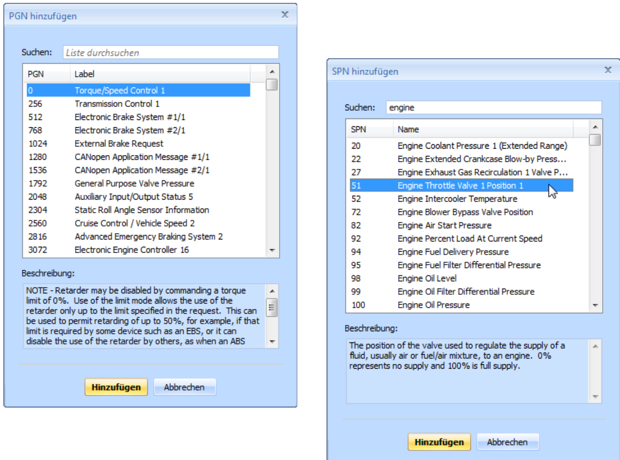
Abbildung 27: SAE J1939 Filterkonfiguration (PGN, SPN)
