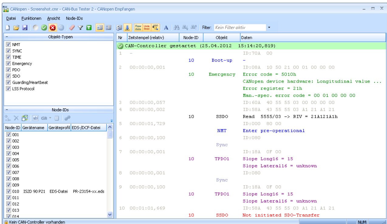
Abbildung 24: Modul: CANopen Empfangen
