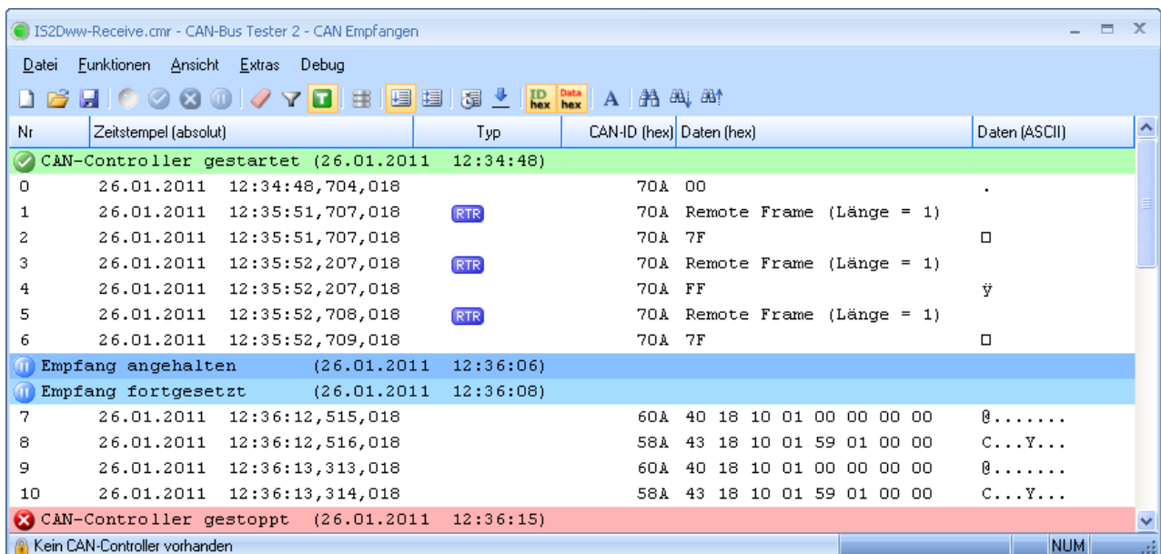
Abbildung 21: Modul: CAN Empfangen - Modus: Scrollen
